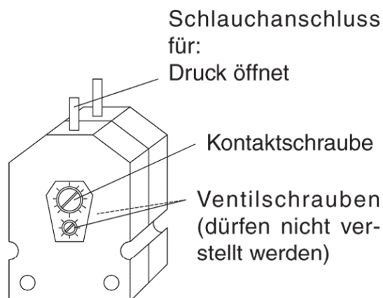
Druckwellenschalter
